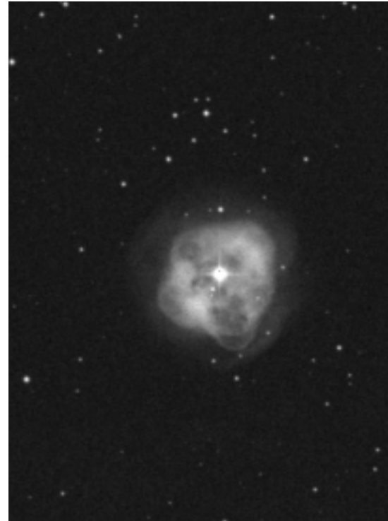
fig. 1 NGC 1514, imagen del DSS. Fue catalogada por Herschel como IV 69
