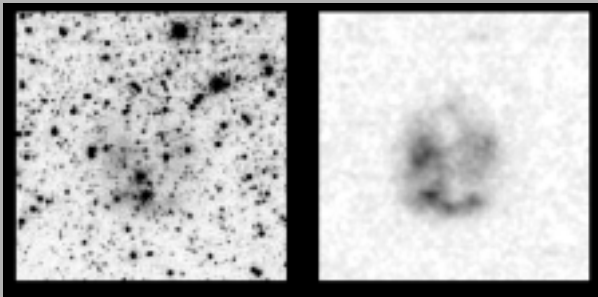
La nebulosa planetaria NGC6441 desde el HST. La imagen de la izquierda es la original y la derecha tiene un procesado especial para resaltar la línea H-Alfa que emite este objeto de 6" de tamaño.
