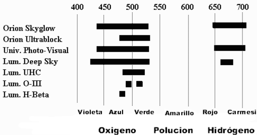
fig. 7. Comparación entre los principales filtros nebulares del mercado. ( www.blackskies.com/tips.html#nebula%20filters )
