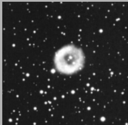
La nebulosa NGC2438, aparentemente dentro de M46 pero físicamente independiente
