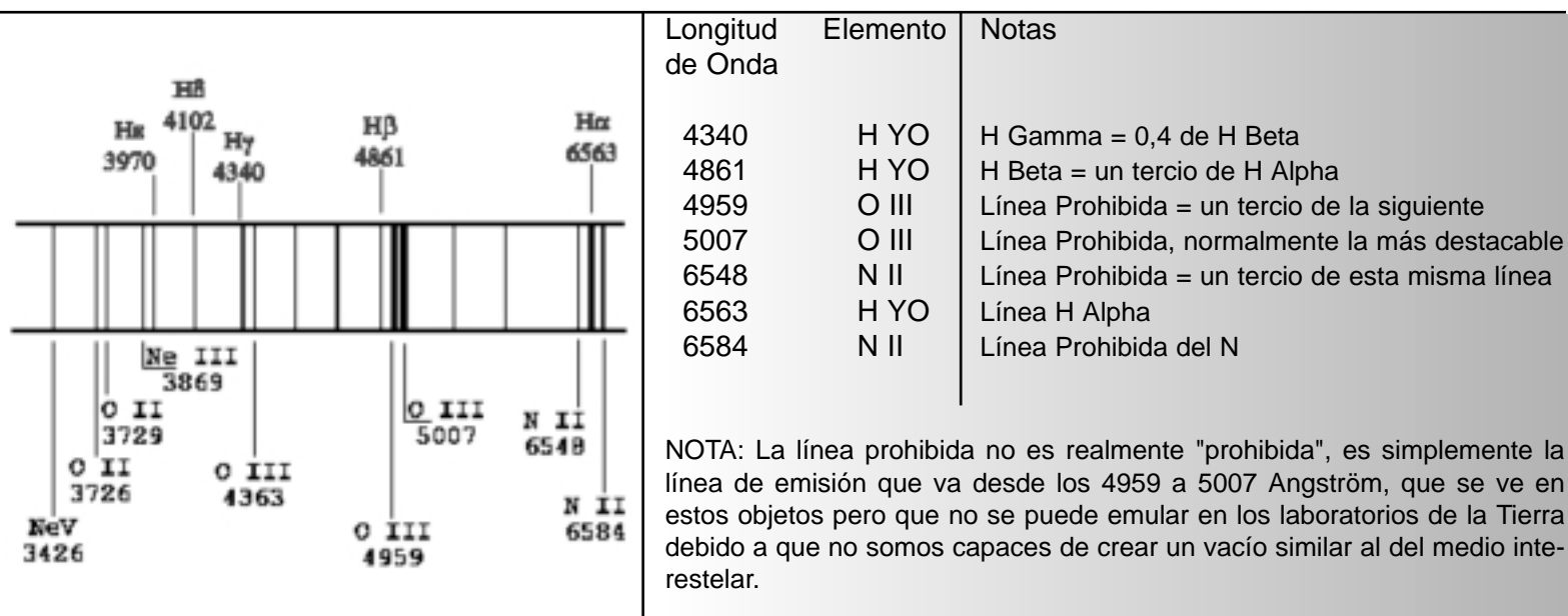
fig. 2 y Tabla I Espectro y líneas de emisión de una nebulosa planetaria. Imagen: http://www.blackskies.com/tips.html#nebula%20filters
