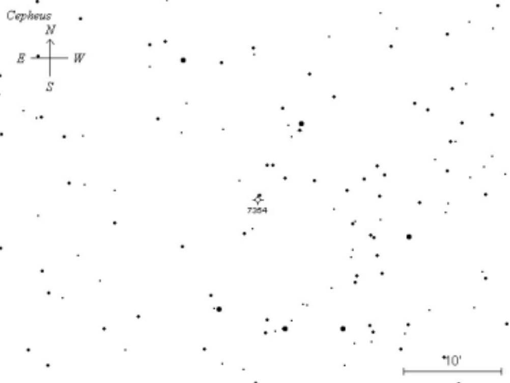
fig 6. Mapa de NGC7354 (obtenido con el Sky Map pro 8)
