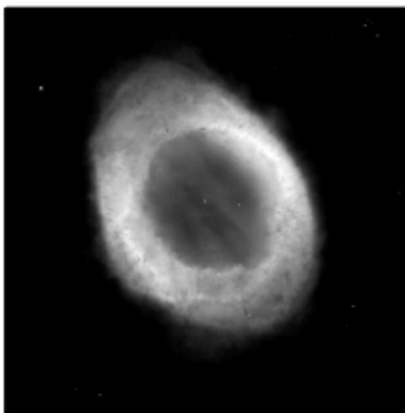
M57, CLASE 4
