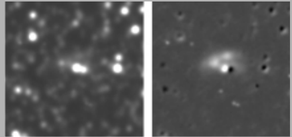
La nebulosa planetaria de M22 desde los observatorios de la Tierra. A la izquierda la imagen original, y a la derecha imagen realzada mediante el contraste con la línea O-III para realzar la emisión del objeto.
