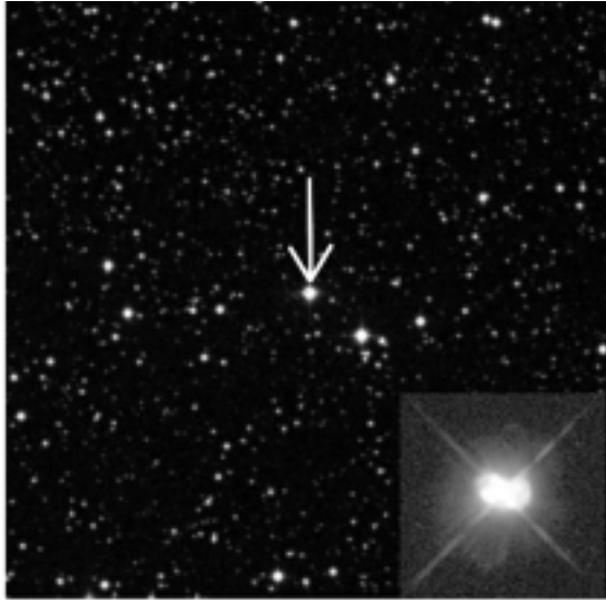
IC4997, CLASE 1
