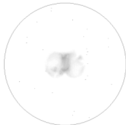
Fig. 8. Comparación del resultado de usar o no filtro nebulares con una nebulosa planetaria. ( www.blackskies.com/images/knisey/m76pn2.gif )
