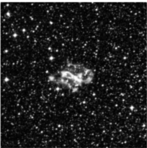
NGC5189, CLASE 5
