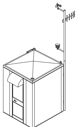
Installazione su cabina Installation on cabin
