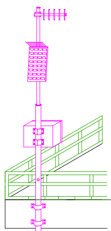
Installazione a muro Installation on wall
