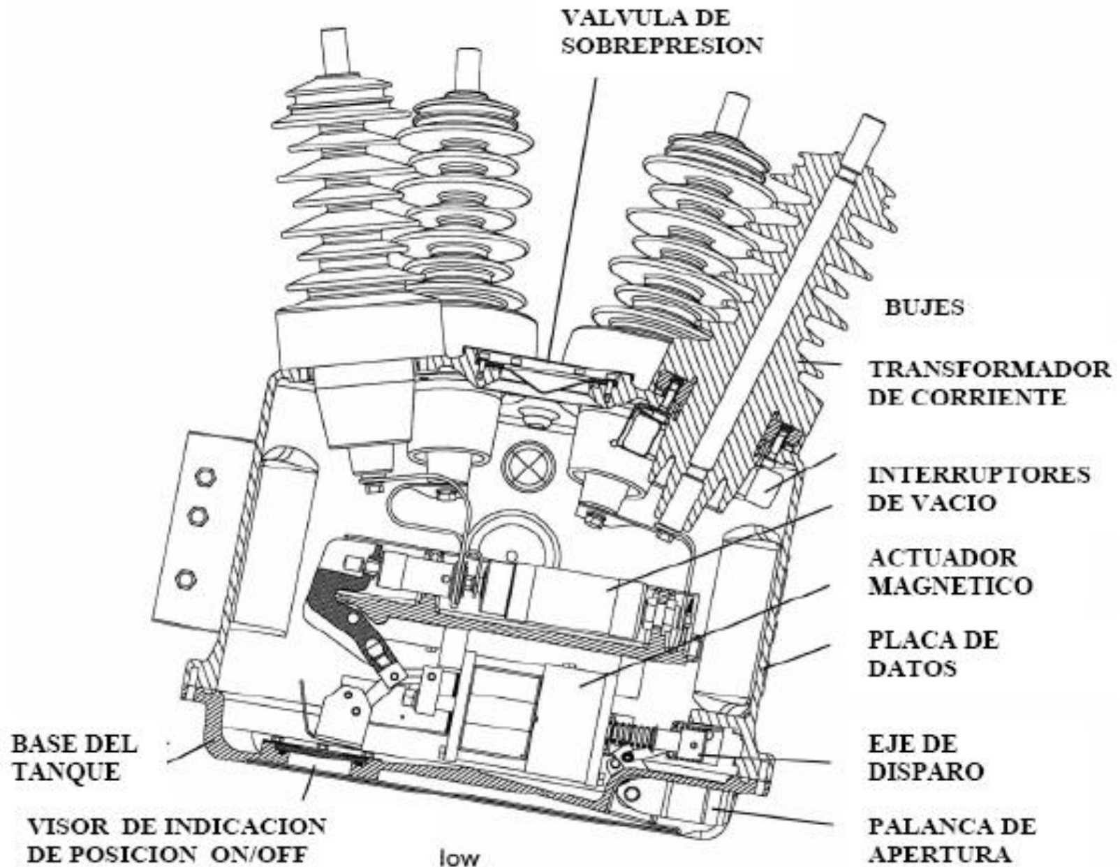
Figura 1: corte lateral del reconectador monofásico de dieléctrico sólido serie W.
