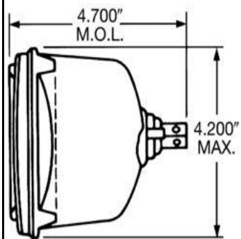
LMP4652 UNIDAD SELLADA 12,8V
